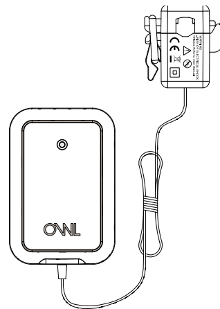
Transmisor con 1 canal (Intensidad máxima 71A – Diámetro del cable 10 mm)
